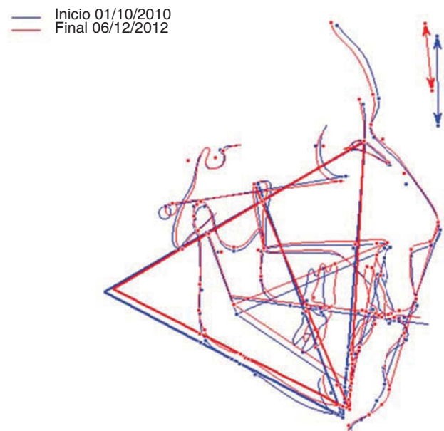
Figura 7. Sobreimposición cefalométrica.
