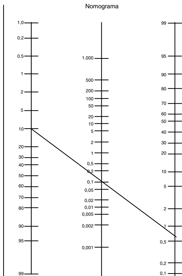
Figura 2 – Normograma de Fagan. Probabilidad pretest y postest para una LR(-) de 0,13.
