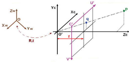
Figura 1. Modelo geométrico de la cámara
