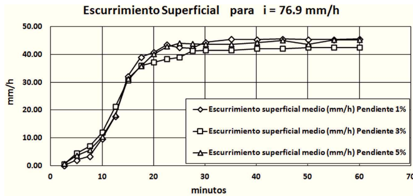
Figura 5. Curvas medias del escurrecimiento superficial en pavimento con diferentes pendientes i = 76.9 mm/h
