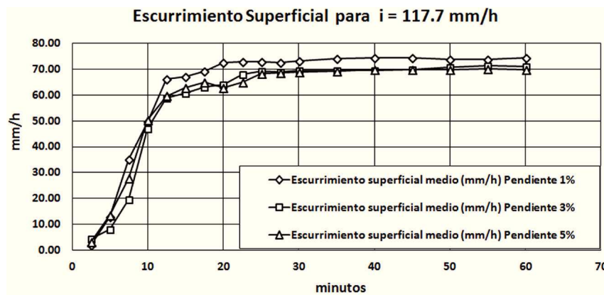
Figura 6. Curvas de las medias del escurrecimiento superficial en pavimento con diferentes pendientes i = 117.7 mm/h
