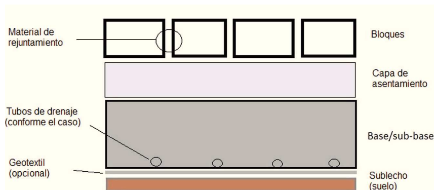
Figura 1. Perfil estándar de un pavimento de bloques intertrabados
