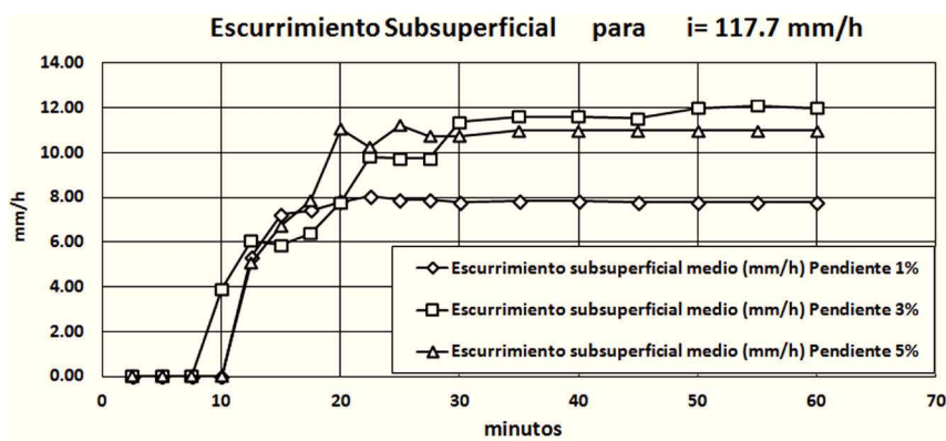
Figura 8. Curvas de las medias del esguerrimiento subsuperficial en pavimento con diferentes pendientes i = 117.7 mm/h
