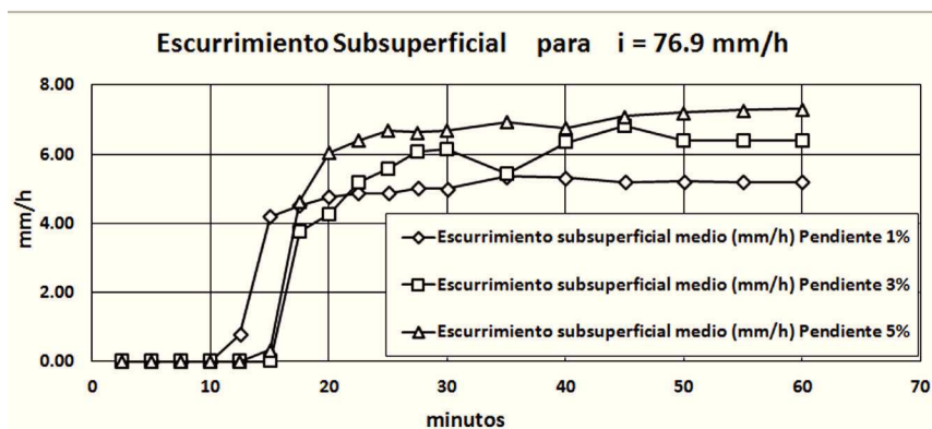
Figura 7. Curvas de las medias del esguerrimiento subsuperficial en pavimento con diferentes pendientes i = 76.9 mm/h
