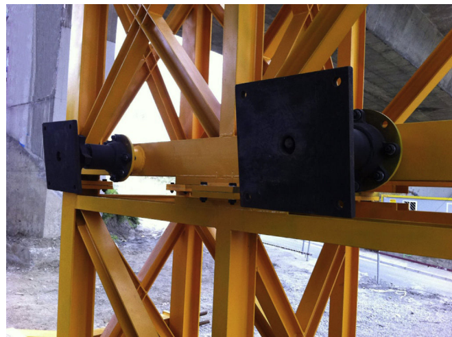
Figura 22. Topes provistos de rótula esférica y husillo de regulación.
