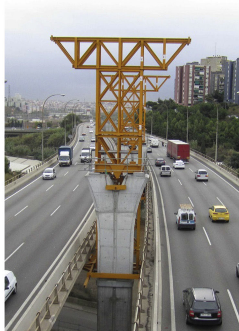
Figura 20. Estructura auxiliar delantera en cabeza de pila. Esquemas y vista frontal real.
