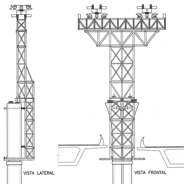
Figura 20. Estructura auxiliar delantera en cabeza de pila. Esquemas y vista frontal real.
