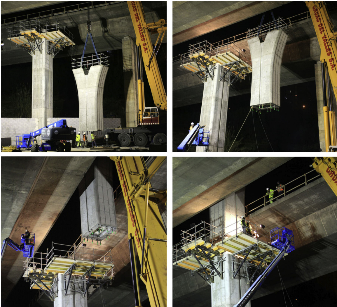
Figura 14. Montaje de la fracción superior de una pila.
