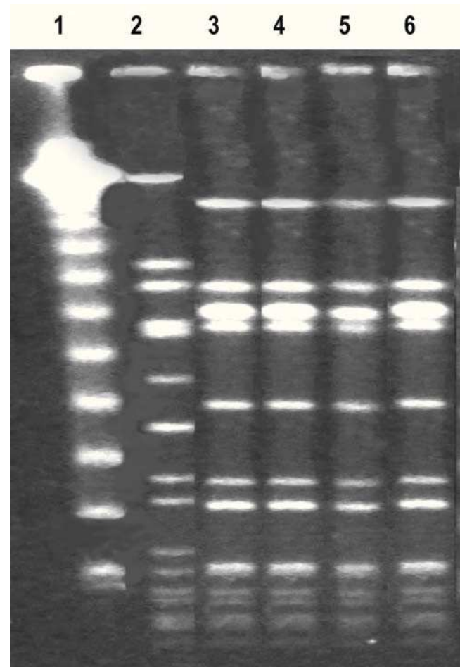
Figura 1 Patrones de SmaI PFGE de los aislamientos SARM-AC 2, 3 y 4. Línea 1: Marcador de peso molecular (Lambda PFG Ladder New England Biolabs); línea 2: NCTC 8325 (cepa de referencia SARM); línea 3: SARM-AC 2 (h-VISA); línea 4: SARM-AC 3 (VISA-NS DAP); línea 5: SARM-AC 4 (VSSA); línea 6: M 2847 [SARM-AC Argentina: ST5 SCCmec IV PVL (+)].
