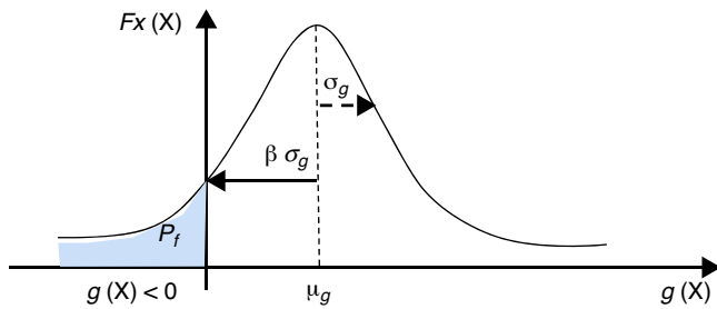
Figura 1. Definição geométrica de confiabilidade.
