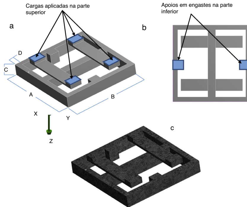
Figura 5. a) Célula de carga para 6 componentes de esforços, b) condição de contorno, c) malha de elementos finitos.
