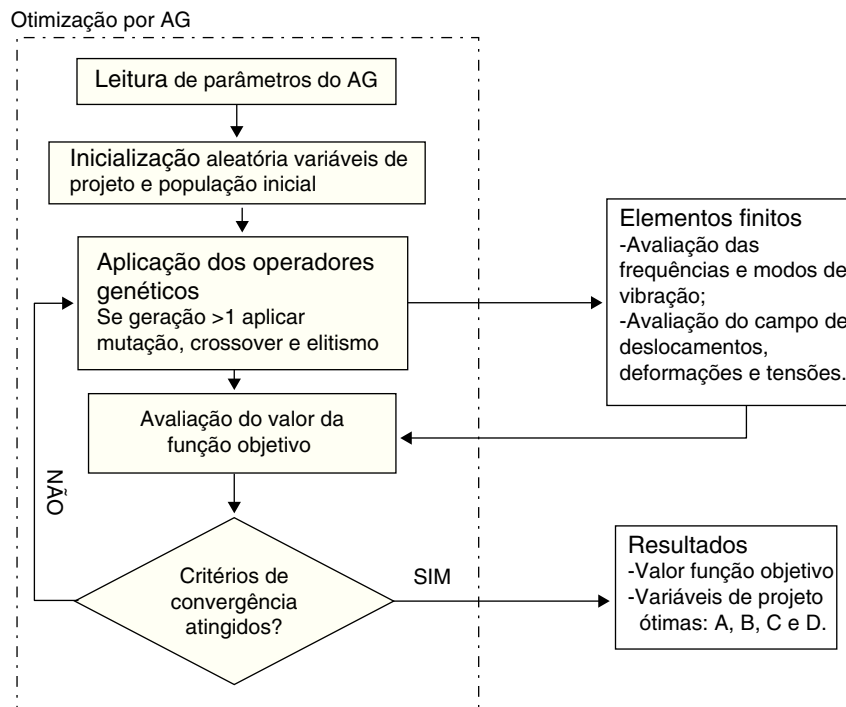
Figura 4. Fluxograma da lógica de otimização (interação entre AG e elementos finitos).
