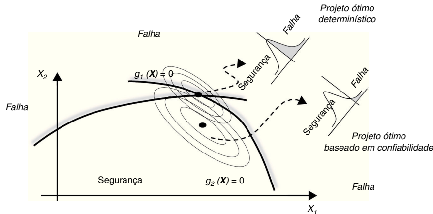
Figura 2. Definição geométrica de otimização determinística e baseada em confiabilidade.
