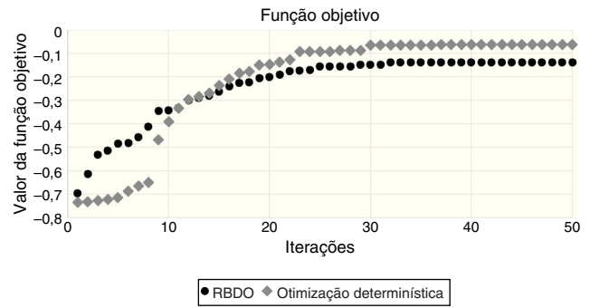
Figura 6. Convergência do valor da função objetivo.
