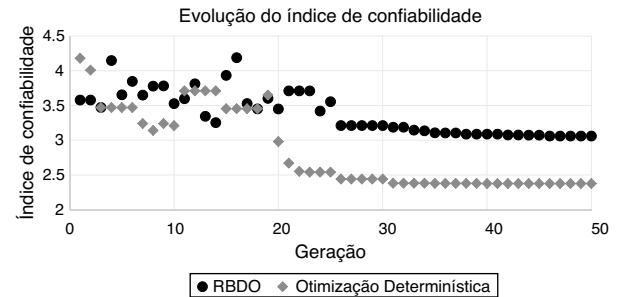
Figura 7. Análise do índice de confiabilidade para cada iteração do AG e da otimização determinística.
