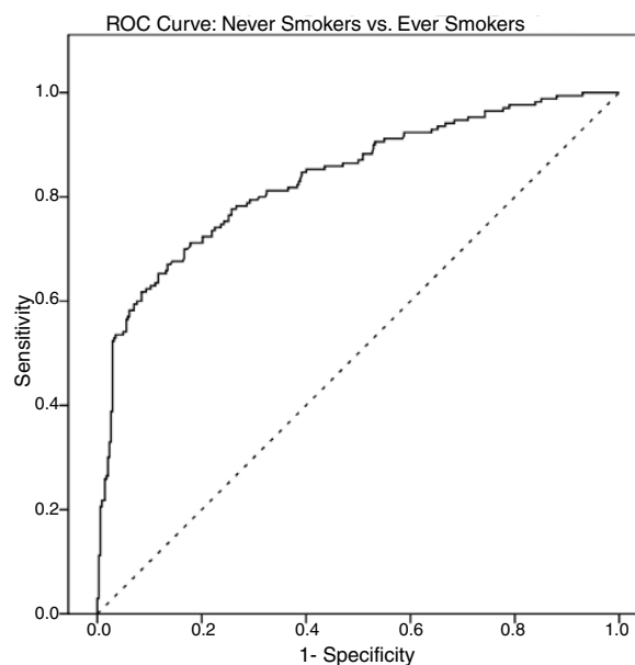
Figura 1 Curva ROC.
