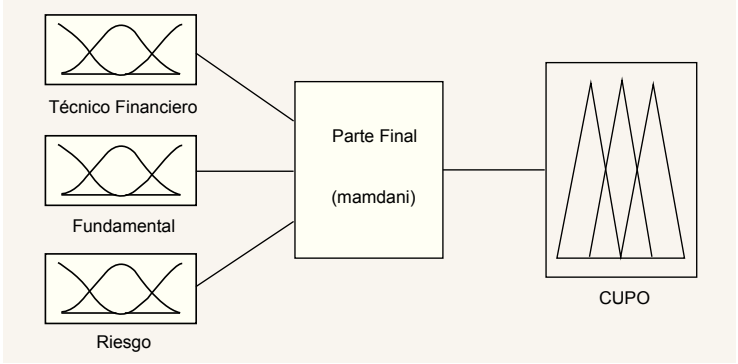
Figura 20. FIS resultado final “cupo”
