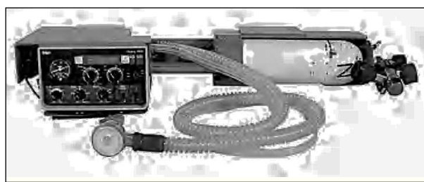
Figura 9. Oxilog 2000.
