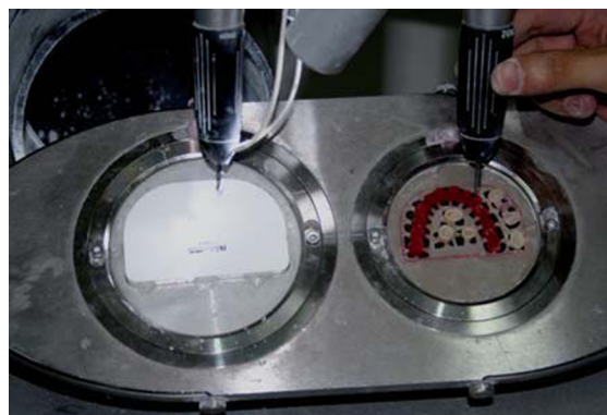
Figura 4. Elaboración de estructura en zirconia.
