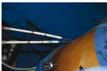
Figura 2 Criosonda de 17Ga del equipo Cryocare Surgical System (Endocare Inc., Irvine, Calif, USA) durante la crioablación renal.
