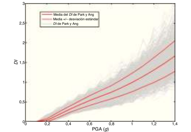
Figura 3. Gráficos de los índices de daño global representados en función de la PGA (curvas de daño), calculados mediante análisis no lineal dinámico para la estructura de la figura 1.
