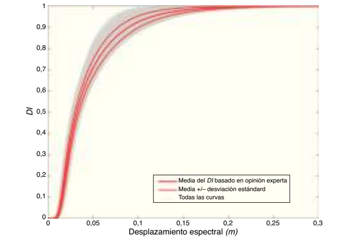
Figura 8. Curvas de vulnerabilidad mostrando los índices de daño representados en función del desplazamiento espectral; los cálculos se han hecho considerando las propiedades mecánicas de los materiales como variables aleatorias.
