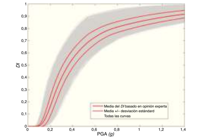
Figura 10. Índices de daños representados en función de la aceleración máxima del terreno. Se han considerado las incertidumbres relacionadas con las propiedades mecánicas de los materiales y con las características de la acción sísmica.
