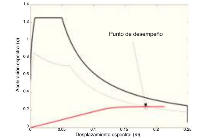
Figura 9. Punto de desempeño para un determinado espectro (método propuesto en el capítulo 8 del ATC-40).
