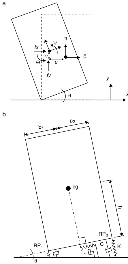
Figura 4. Modelo de Elemento Rígido y Resortes: a) sistema de referencia; b) resortes y amortiguadores.
