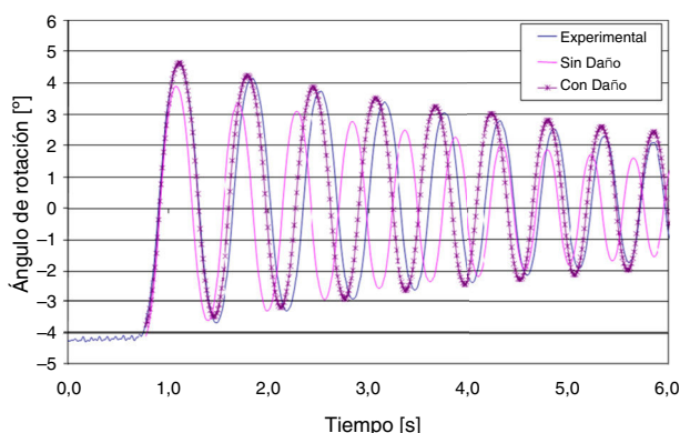
Figura 9. Balanceo libre de un cuerpo rígido dañado.
