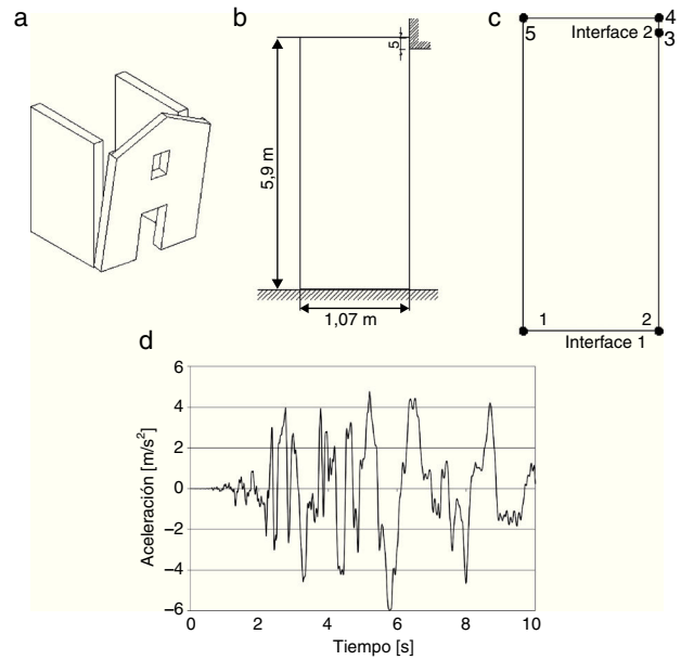
Figura 10. Ejemplo de un cuerpo rígido con asimetría de frontera: a) muro de mampostería separada del resto de la estructura; b) dimensiones; c) modelo e interfaces; d) registro sísmico.
