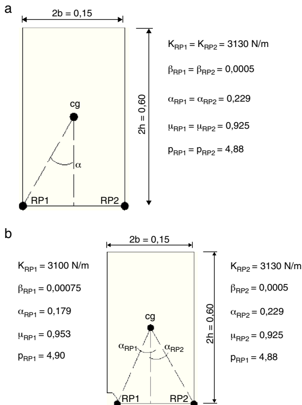
Figura 8. Geometría y propiedades de un cuerpo rígido rectangular con asimetría de base: a) bloque sin daño; b) bloque con daño.
