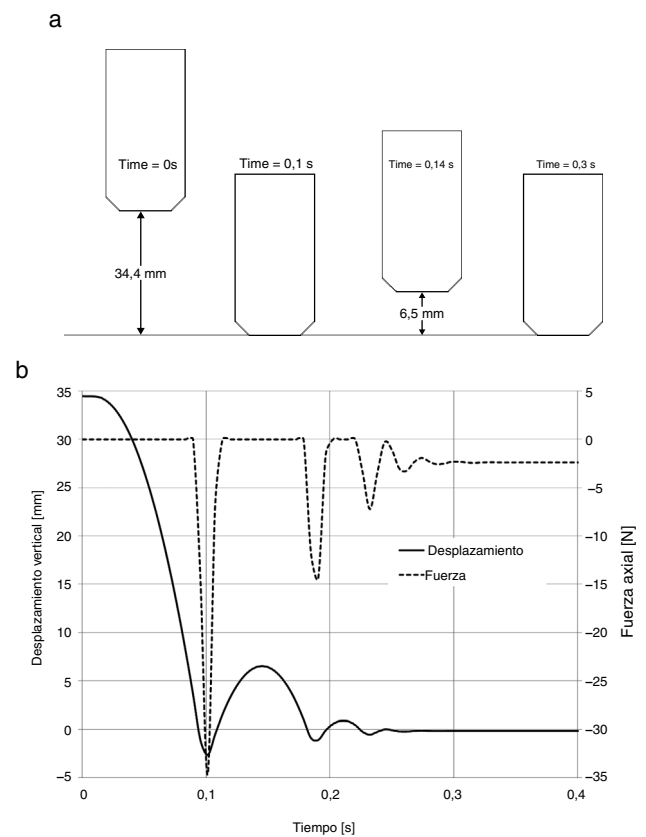
Figura 7. Respuesta típica de un bloque rígido en caída libre: a) representación esquemática de la prueba a diferentes tiempos; b) desplazamientos verticales y fuerzas axiales en los resortes.
