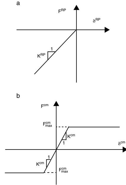
Figura 5. Leyes constitutivas de los resortes: a) axial; b) cortante.
