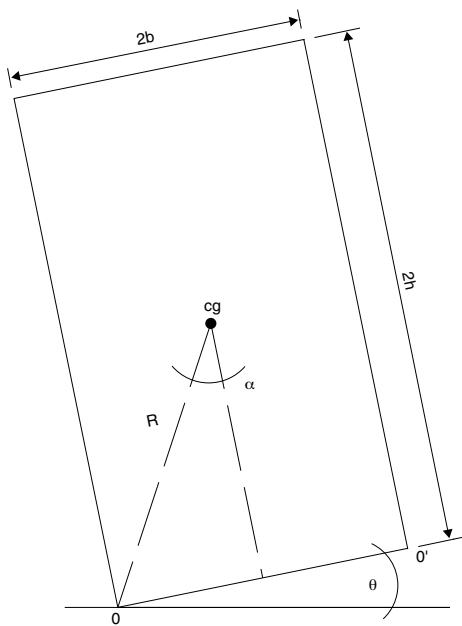
Figura 3. Esquema de un bloque rígido.
