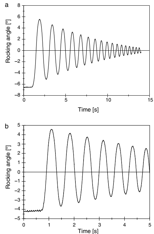
Figura 1. Respuestas típicas de bloques rígidos a balanceo libre: a) balanceo simétrico; b) balanceo asimétrico [24].
