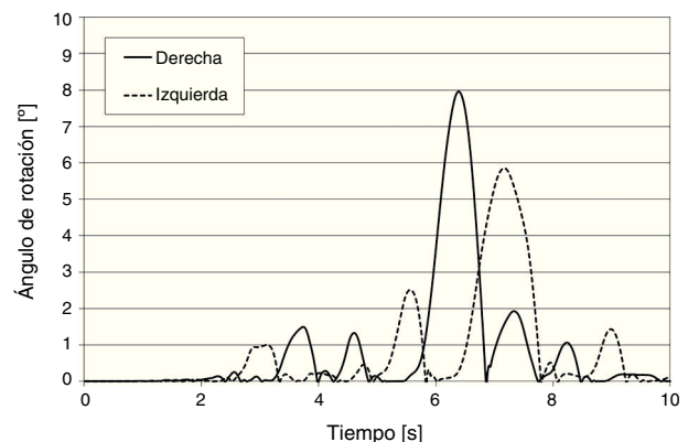
Figura 11. Respuesta típica de un bloque con asimetría de frontera sometido a un registro sísmico real.
