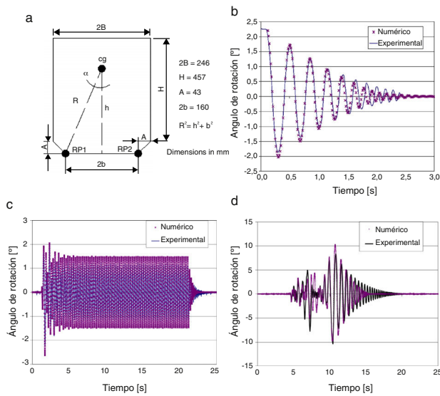
Figura 6. Respuesta típica de un bloque rígido ante diferentes tipos de movimiento: a) geometría del bloque; b) balanceo libre; c) movimiento armónico (seno con una frecuencia de 4 Hz y 4 mm de amplitud); d) movimiento aleatorio.
