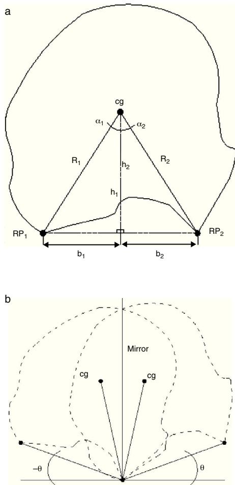
Figura 2. Simetría dinámica: a) cuerpo asimétrico con simetría dinámica; b) simetría de los puntos de rotación [27].
