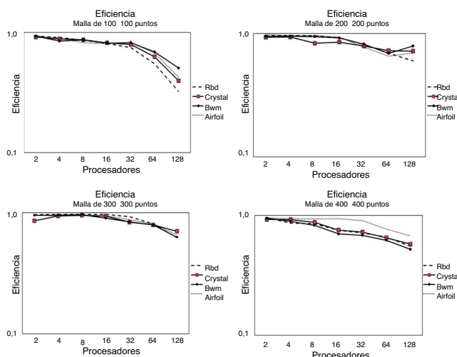
Figura 2. Eficiencia de la implementación (mostrada en escala logarítmica) aumentando la cantidad de puntos en las mallas: a) 100 × 100; b) 200 × 200; c) 300 × 300; d) 400 × 400.
