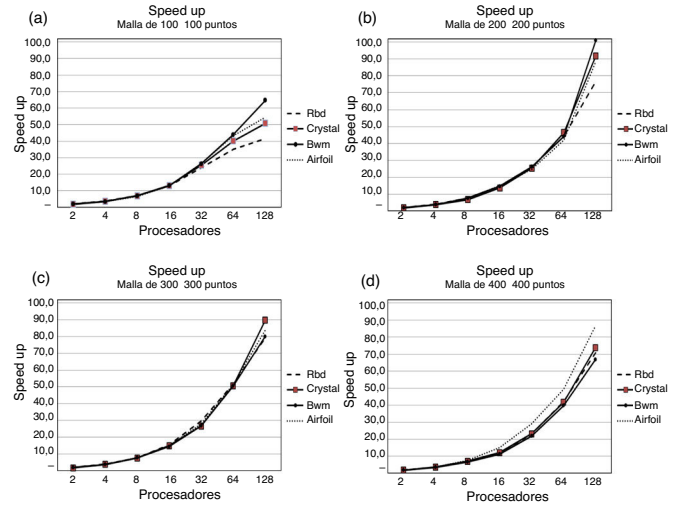
Figura 1. Speedup obtenido al aumentar la cantidad de puntos en las mallas: a) 100 \times 100 ; b) 200 \times 200 ; c) 300 \times 300 ; d) 400 \times 400 .
