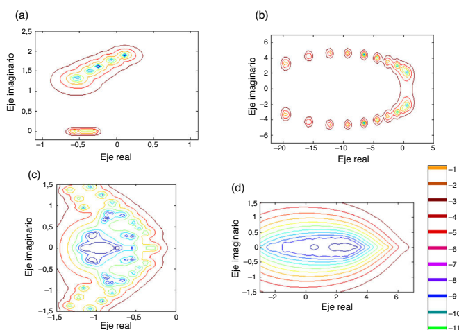
Figura 3. Pseudoespectro de las matrices: a) Rdb; b) Bwm; c) Airfoil; d) Crystal para \epsilon = 10^{-1}, 10^{-2}, \dots, 10^{-11} .
