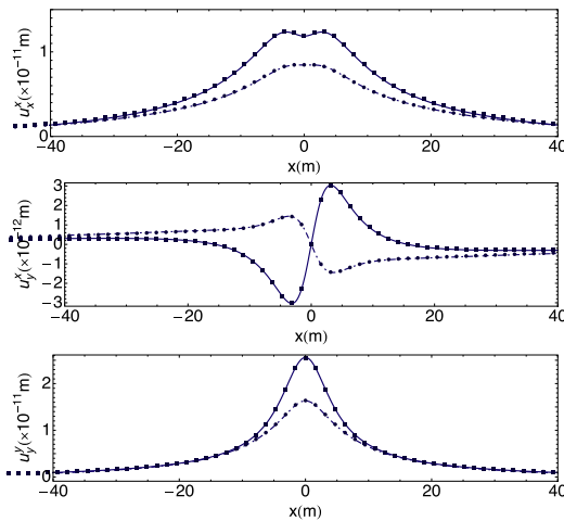
Figura 8. Desplazamientos en la superficie (línea continua y puntos) y sobre la línea y = -h (línea discontinua y puntos) debido a una carga unitaria aplicada en el origen obtenida con la SF de Mindlin (líneas) [12] y calculada mediante la transformada de la SF (puntos).
