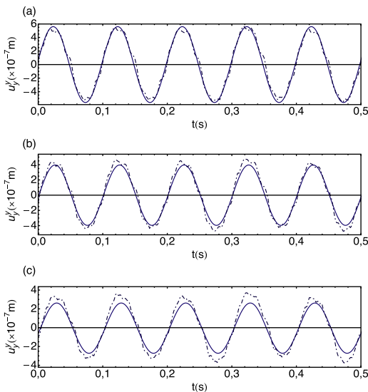
Figura 6. Desplazamiento vertical debido a una carga armónica de 402 N y 10 Hz aplicada en la superficie de un semiespacio, obtenida mediante datos experimentales (línea discontinua) y calculada mediante la transformada inversa de Fourier de la SF (línea continua): (a) 1,0 m, (b) 1,5 m, (c) 2,0 m.
