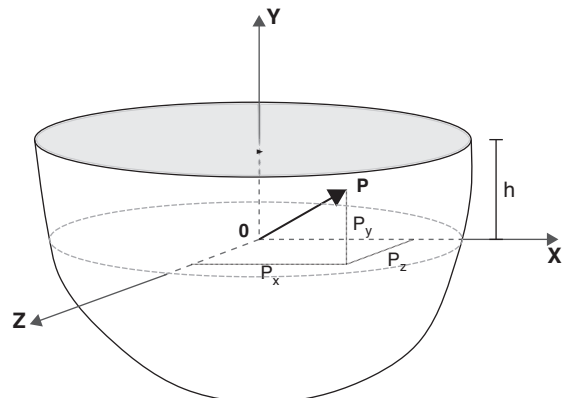
Figura 1. Semiespacio bajo carga puntual.
