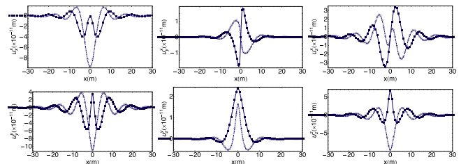
Figura 7. Componentes real (línea continua y puntos sombreados) e imaginaria (línea discontinua o puntos) del desplazamiento sobre la línea y=1 debido a una carga armónica unitaria \omega=100 Hz aplicada en el origen obtenida a partir de la SF 2.5D para el espacio completo (líneas [22]) y calculada mediante la transformada inversa de Fourier en k_x de la SF transformada (cuadrados); en todos los casos k_z=0,5 .
