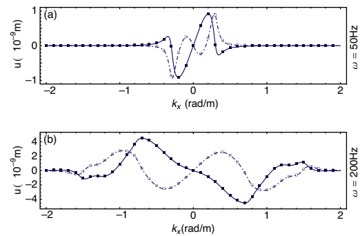
Figura 3. Validación del teorema de reciprocidad. Parte real (línea continua) e imaginaria (línea discontinua) de u_z^x ; parte real (cuadrado sombreado) e imaginaria (cuadrado de líneas de puntos) de u_x^z .
