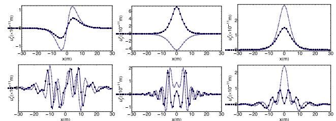
Figura 4. Partes real (línea continua o cuadrado sombreado) e imaginaria (línea discontinua o cuadrado) para los desplazamientos sobre la línea ( y=5 ) debido a una carga unitaria y armónica de 50 Hz (arriba) y 200 Hz (abajo) aplicada en el origen, obtenida mediante el Método de Elementos de Contorno (líneas) y calculada mediante la transformada inversa de Fourier en k_x de la solución fundamental (punteada); número de onda k_z = 0,5 en todos los casos.
