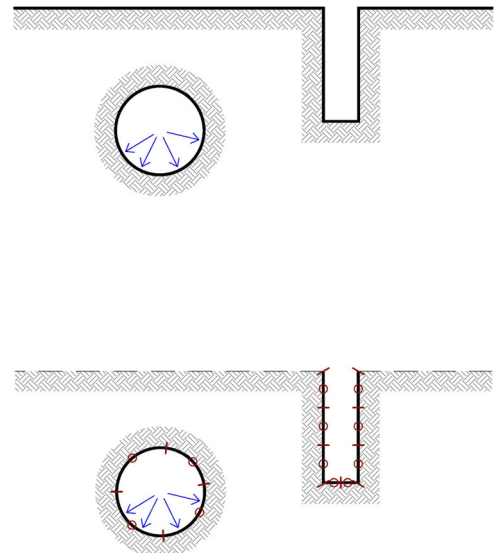
Figura 10. Problema dinámico 2.5D en un semiespacio.
