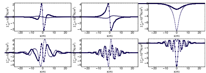
Figura 5. Partes real (línea continua o cuadrado sombreado) e imaginaria (línea discontinua o cuadrado) para las tensiones sobre la línea ( y=2 ) debido a una carga unitaria y armónica de 50 Hz (arriba) y 200 Hz (abajo) aplicada en el origen, obtenida mediante el Método de Elementos de Contorno (líneas) y calculada mediante la transformada inversa de Fourier en k_x de la solución fundamental (punteada); número de onda k_z = 0,5 en todos los casos.
