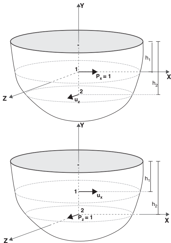
Figura 2. Comparación de reciprocidad.
