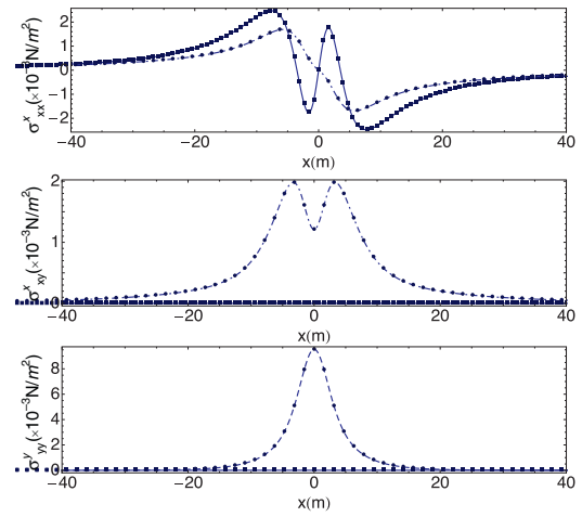
Figura 9. Tensiones en la superficie (línea continua y puntos) y sobre la línea y = -h (línea discontinua y puntos) debido a una carga unitaria aplicada en el origen obtenida con la SF de Mindlin (líneas) [12] y calculada mediante la transformada de la SF (puntos).
