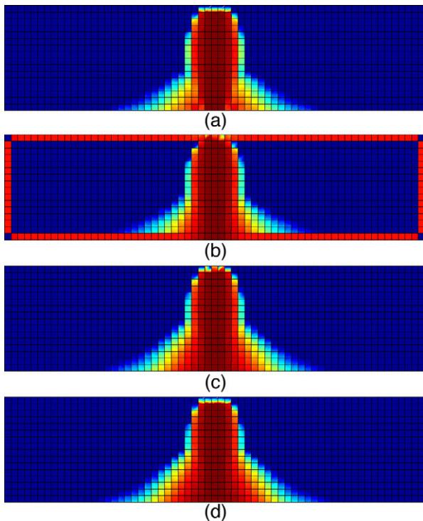
Figura 8. Ensayo de flexión en tres puntos: campos de daño obtenidos mediante condiciones de contorno (a) de Dirichlet, (b) de Neumann homogéneas, (c) de Neumann no homogéneas y (d) combinadas.
