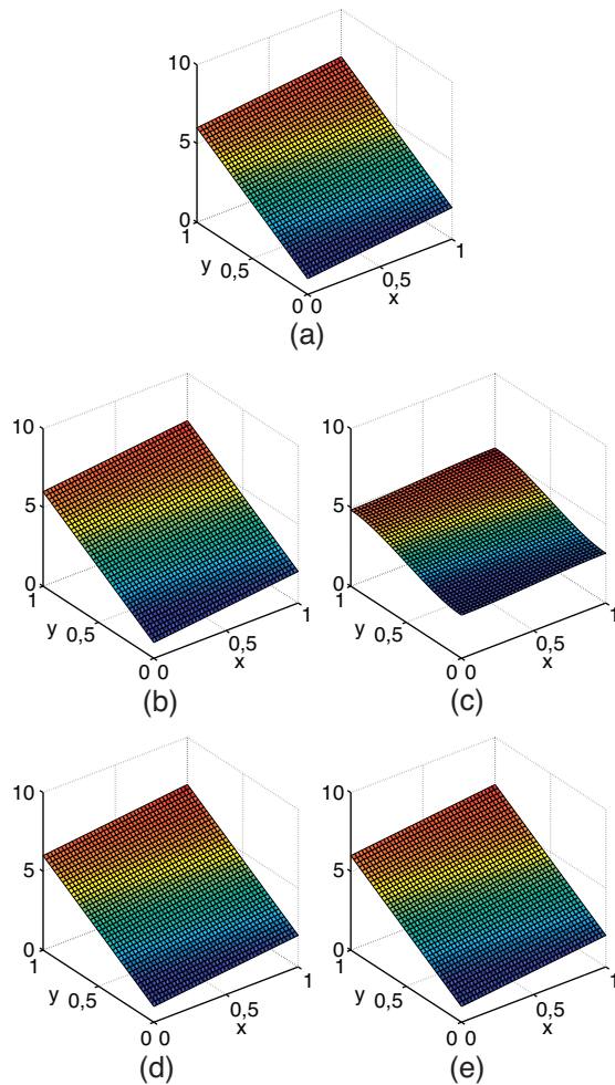
Figura 1. Test de validación con (a) u(\mathbf{x})=u(x, y)=1+x+5y . Soluciones \tilde{u} , donde \tilde{\mathbf{u}}=(\tilde{u}_x, \tilde{u}_y) , obtenidas al imponer condiciones de contorno (b) de Dirichlet, (c) de Neumann homogéneas, (d) de Neumann no homogéneas y (e) combinadas.
