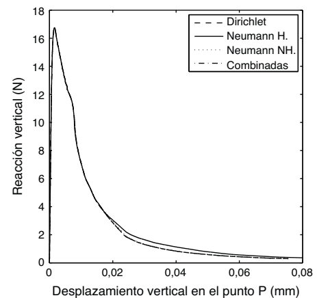
Figura 10. Ensayo de tracción directa: curvas fuerza-desplazamiento.
