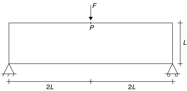
Figura 6. Ensayo de flexión en tres puntos: planteamiento del problema.
