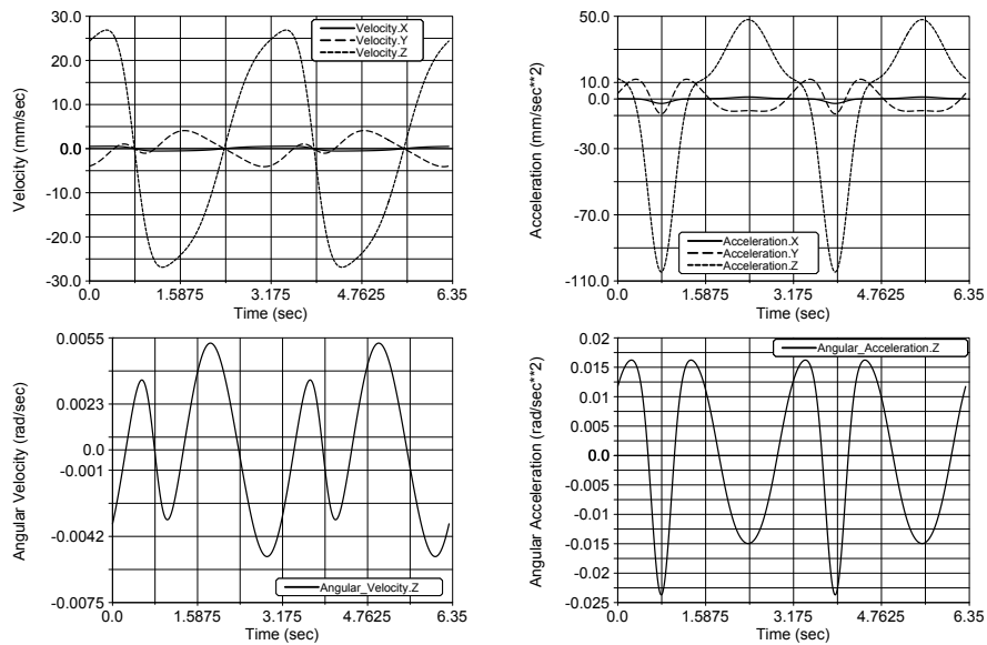
Figura 9: Cinemática infinitesimal del manipulador usando ADAMS
