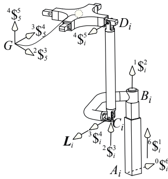
Figura 3: Singularidad estructural: {}^3S_i^4 y {}^5S_i^6 son concurrentes.
