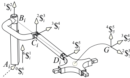
Figura 4: Singularidad inversa: B_i , C_i y D_i son colineales
