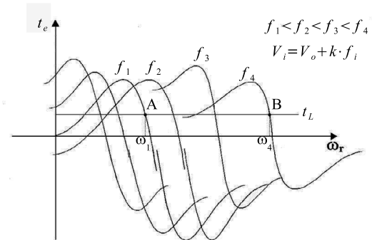
Figura 1: Curvas de funcionamiento del motor de inducción para distintas frecuencias de alimentación
