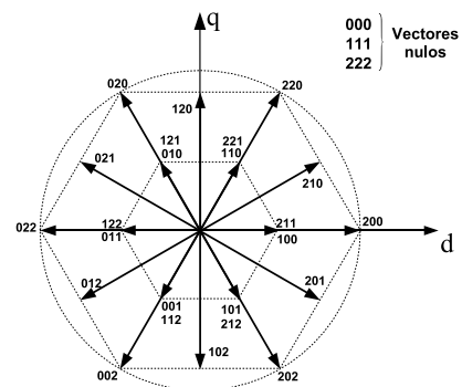
Figura 7: Vectores disponibles en un inversor de tres niveles
