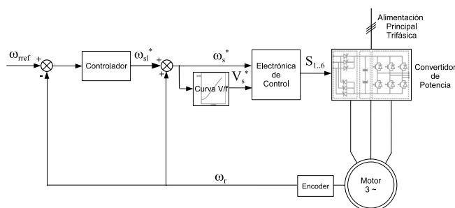
Figura 2: Esquema general del control Tensión-Frecuencia
