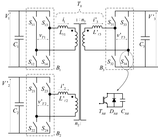
Figura 1: Topología del CTP
