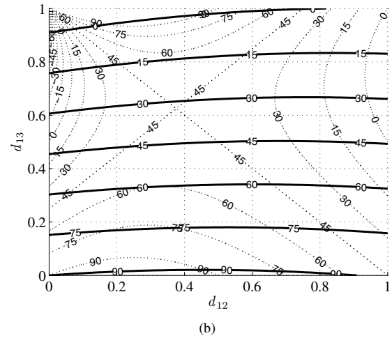
Figura 6: Desfases límites en el plano d_{13} vs. d_{12} a partir del cual el CTP opera con conmutación suave: (a) \delta_{12} y (b) \delta_{13} .
