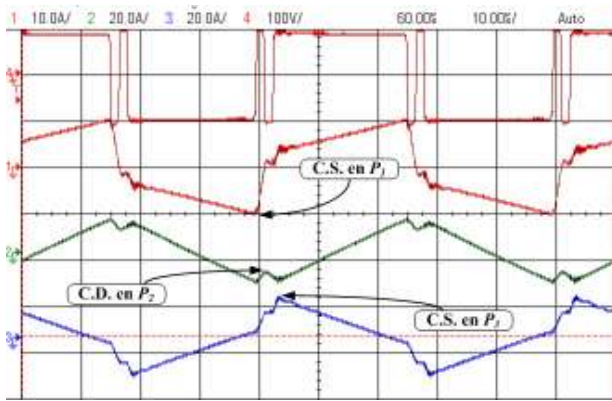
Figura 8: Formas de onda experimentales para una operación con conmutación dura.
