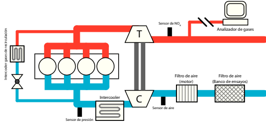
Figura 4: Esquema del motor con los principales sensores instalados, destacando especialmente el sensor de NO x en el escape del mismo.
