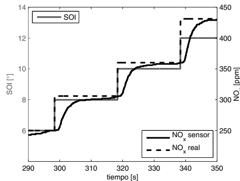
Figura 1: Respuesta de un sensor de \text{NO}_x -curvas negro y eje derecho- a escalones de avance en la inyección (SOI)-curva gris y eje izquierdo-. La medida de \text{NO}_x presenta una clara respuesta dinámica con respecto a la señal de actuación de SOI. La respuesta dinámica puede ser ajustada con un filtro de primer orden y un retraso. En la figura, se indica asimismo la respuesta real esperada (Galindo et al., 2011), cuyo valor se pretende estimar en el presente artículo. Las unidades de SOI son grados de cigüeñal antes del punto muerto superior [°], mientras que los \text{NO}_x son medidos en ppm. El retraso está en el orden de 1 s mientras que el tiempo de respuesta está en torno a 0.75 s.
