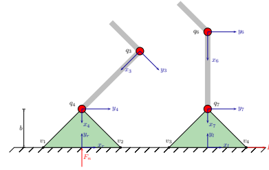
Figura 6: Pies del robot
