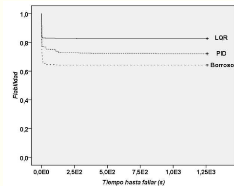
Figura 12: Curvas de fiabilidad de los representantes de los controladores LQR, PID y borroso con dos defectos inyectados.
