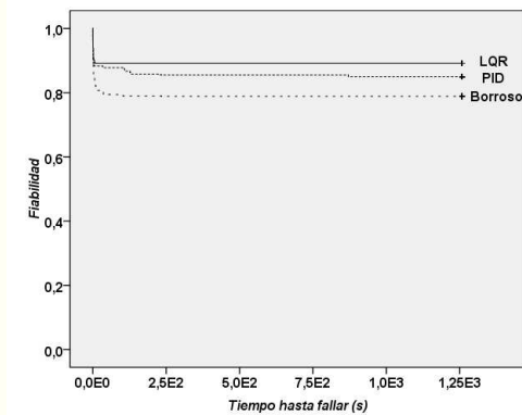
Figura 11: Curvas de fiabilidad de los representantes de los controladores LQR, PID y borroso con un defecto inyectado.
