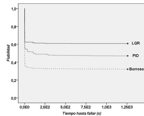
Figura 15: Curvas de fiabilidad de los representantes de los controladores LQR, PID y borroso con cinco defectos inyectados.
