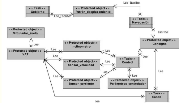
Figura 9: Perspectiva más detallada de los componentes de una simulación
