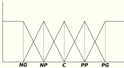
Figura 4: Patrón de funciones de pertenencia para señales de entrada y salida.
