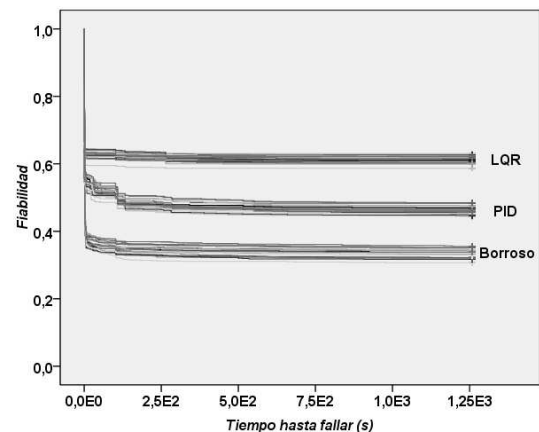
Figura 10: Curvas de fiabilidad de 30 controladores LQR (arriba), 30 controladores PID (en medio) y 30 controladores de tipo borroso (abajo).
