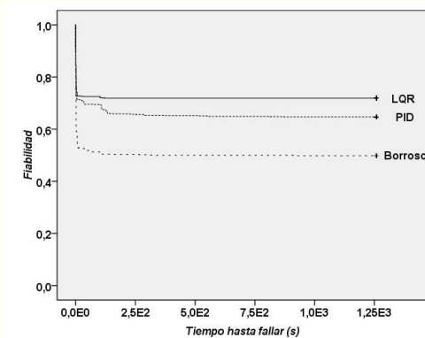
Figura 13: Curvas de fiabilidad de los representantes de los controladores LQR, PID y borroso con tres defectos inyectados.
