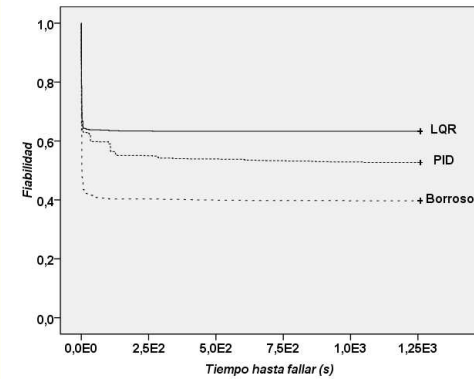
Figura 14: Curvas de fiabilidad de los representantes de los controladores LQR, PID y borroso con cuatro defectos inyectados.
