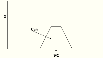
Figura 5: Ejemplo de triángulo truncado correspondiente a la función de pertenencia de la etiqueta de salida C_o , en donde C_{alt} se calcula según (9).
