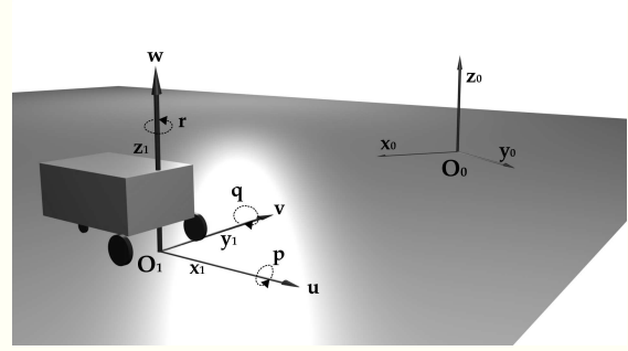
Figura 2: Representación de los marcos de referencia local y global.
