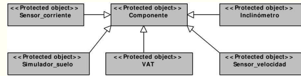
Figura 7: Componentes electromecánicos y simulador del suelo obtenidos por medio de herencia.
