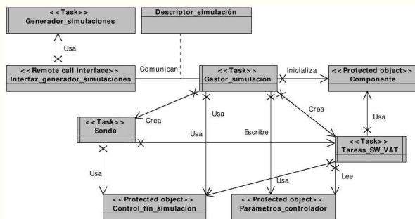
Figura 6: Componentes fundamentales del sistema multicomputador que ejecuta el AG de ajuste de controladores.
