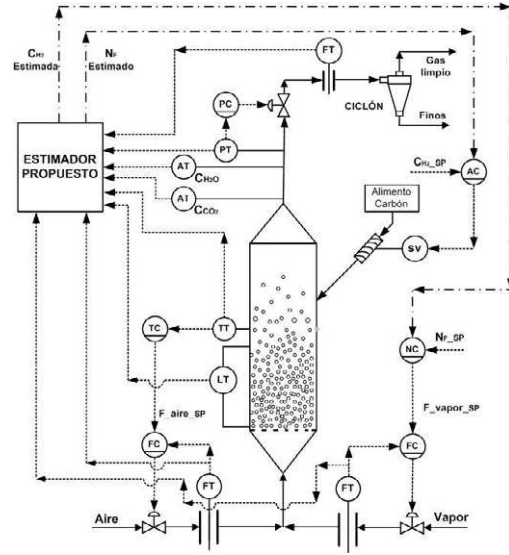
Figura 3: Esquema del GCLF controlado
