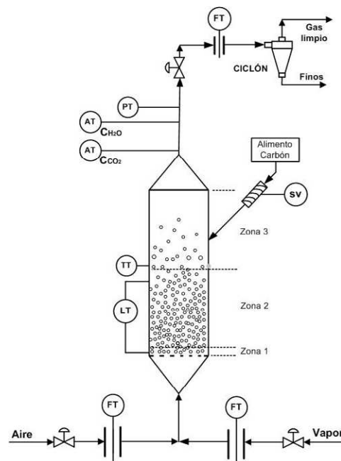
Figura 1: Esquema del gasificador de carbón en lecho fluidizado
