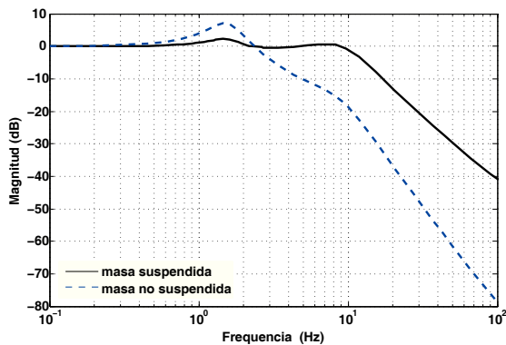
Figura 6: Respuesta en frecuencia del sistema.
