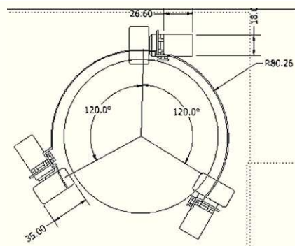
Figura 5: Estructura Robótica con sus ruedas colocadas cada 120 grados.
