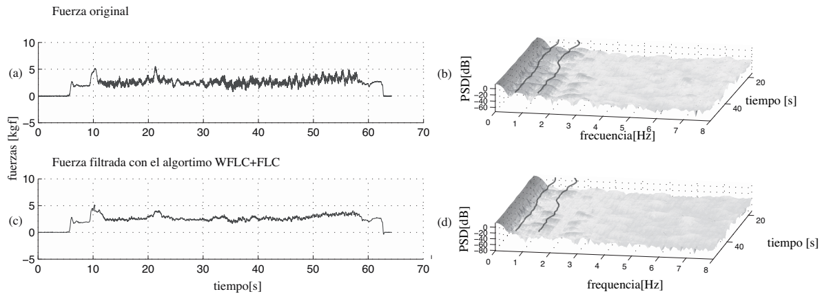
Figura 13. (a) Fuerza medida en el eje Y del sensor de fuerza derecho. Entrada del algoritmo de filtrado. (b) Espectrograma de las señal de fuerza original. (c) Salida del algoritmo de filtrado WFLC-FLC desarrollado en este trabajo y su correspondiente (d) espectrograma. En ambos espectrogramas las líneas continuas se corresponden a la evolución temporal de los los dos armónicos sobre los cuales se aplica el filtrado adaptativo.
