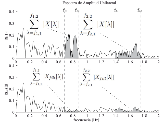
Figura 12. Representación gráfica de los términos utilizados para el cálculo del índice R . En este ejemplo, f_{1,1} = 6,87 \cdot 10^{-1} , f_{1,2} = 8,76 \cdot 10^{-1} , f_{2,1} = 1,38 \cdot 10^{-1} y f_{2,2} = 1,75 \cdot 10^{-1} .
