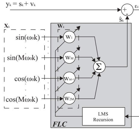
Figura 10. El algoritmo FLC. Este algoritmo adaptativo compone una serie dinámica de Fourier truncada para modelar la señal de entrada, conociéndose la frecuencia de esta señal.
