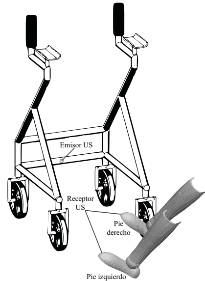
Figura 2. Detalle del subsistema ultrasónico para la medición de la evolución de los pies.
