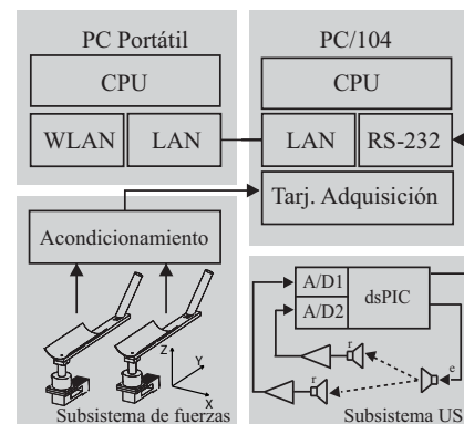
Figura 3. Arquitectura electrónica implementada y utilizada en este trabajo.
