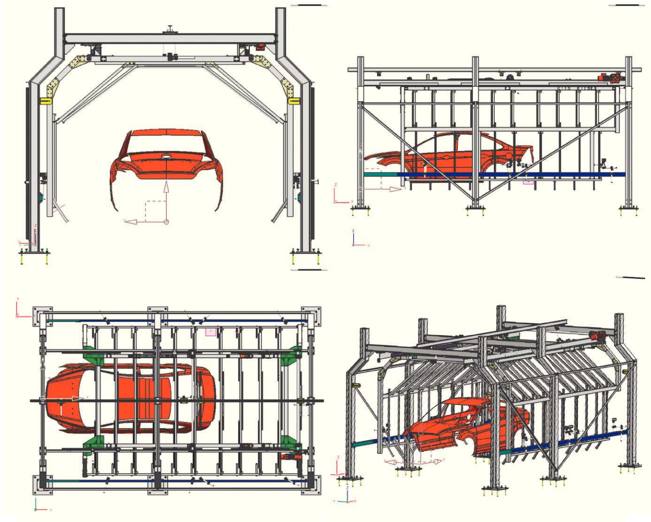
Figura 7: Vistas del túnel de inspección diseñado.
