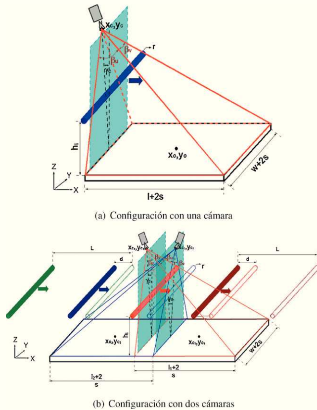
Figura 5: Configuración de las cámaras e iluminación.
