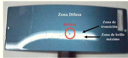
Figura 2: Reflejo basado en tubo fluorescente de alta frecuencia sobre superficie metálica especular y defecto marcado en rojo.
