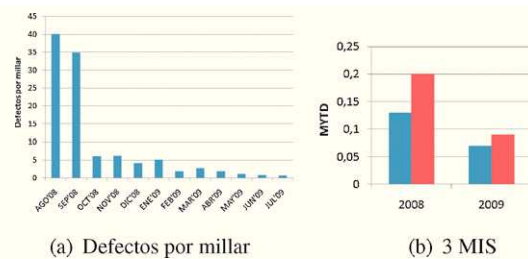
Figura 13: Número de defectos por millar no detectados, medidos a la salida de la factoría y Media anual de reclamaciones post-venta por millar durante los primeros 3 meses en servicio (MIS).
