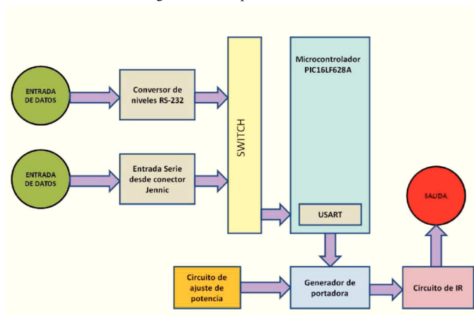
Figura 3: Diagrama de bloques del emisor de infrarrojos.
