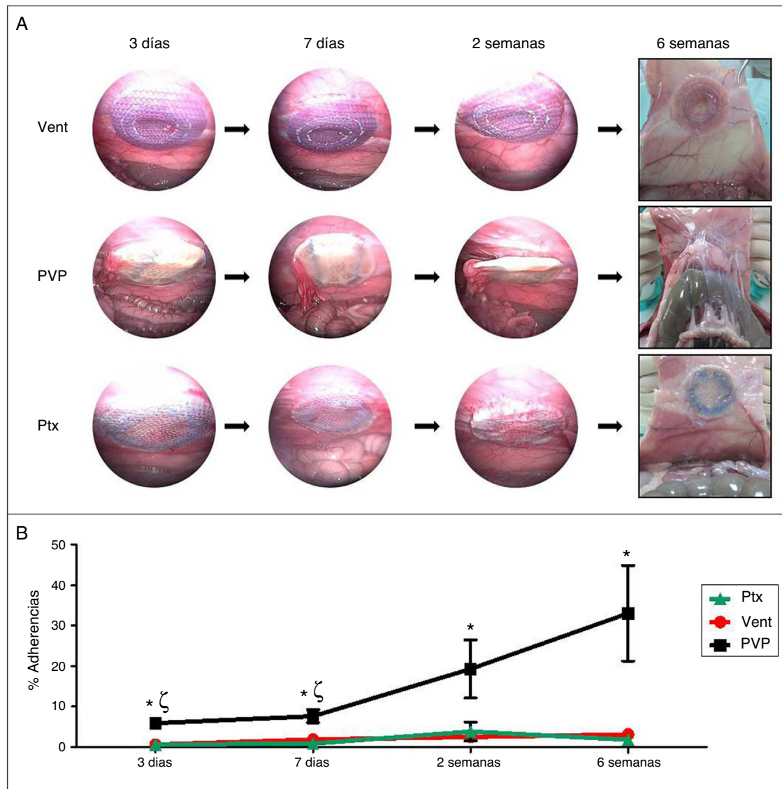
Figura 2 – A) Laparoscopia secuencial; B) Porcentaje de adherencias (*p < 0.05 respecto a VL y Ptx; ζ p < 0.05 respecto a PVP en 6 semanas).
