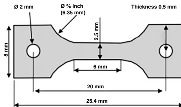
Figura 1 Geometría de forma de hueso de perro utilizada en la fabricación de las probetas.
