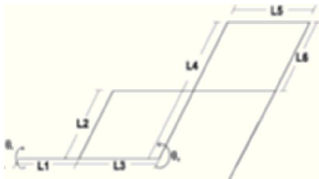
Figura 1. Implementación del punto fijo mediante sistema de barras en configuración de paralelogramo.
