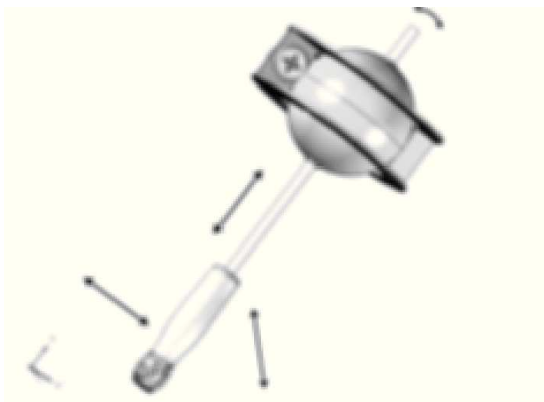
Figura 3. Implementación del punto fijo mediante sistema mecánico en configuración de articulación esférica.
