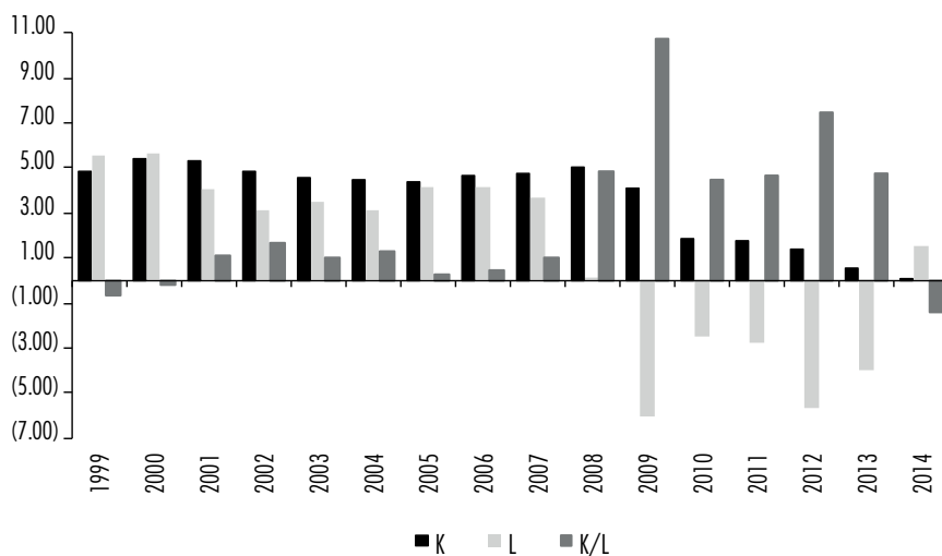
Gráfica 1. Tasas de variación anual del ratio capital-trabajo y sus determinantes (%)
