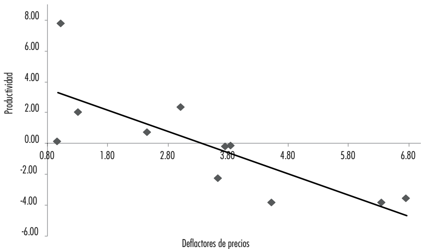
Gráfica 5. Deflatores de precio y productividad por sector de actividad Series en porcentaje para el periodo 1999-2007
