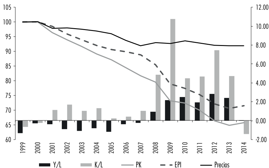
Gráfica 3. Ratio producto-capital y sus determinantes, la eficiencia productiva de la inversión y el ratio de precios (1999= 100)
