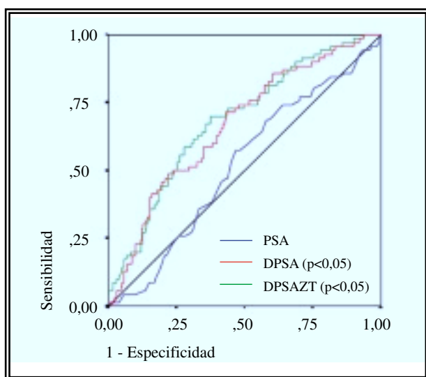
FIGURA 1. Curvas del rendimiento diagnóstico para el PSA, PSA densidad (DPSA) y PSA densidad de la zona de transición (DPSAZT) para toda la muestra.
