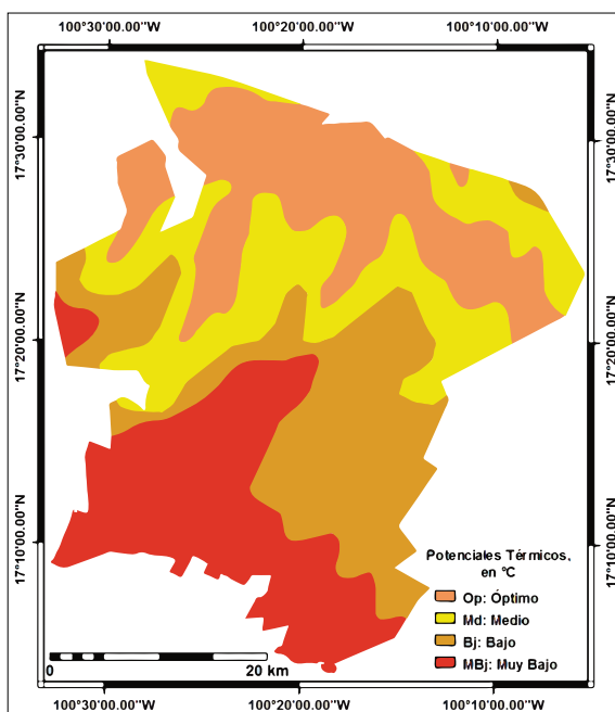
Figura 5. Potenciales térmicos, en °C.
