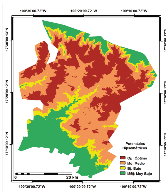
Figura 2. Potenciales hipsométricos para el cultivo del café.
