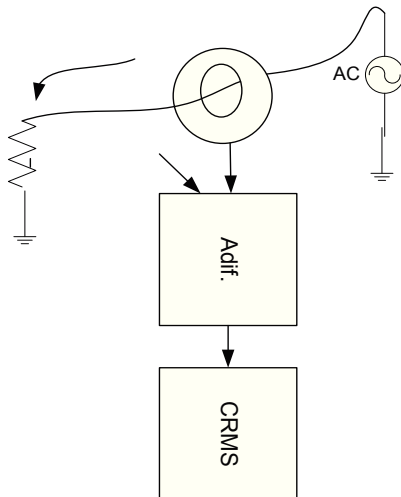
Figura 19. Bosquejo de la medición de corriente de 120 Vca a 60 Hz utilizando el "Wathorímetro K0", con un transformador toroidal de corriente de 20 Amperios como sensor
