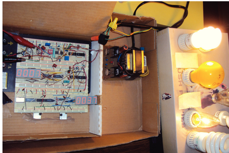
Figura 20. Maqueta del "Wathorímetro K0" en operación, mostrando el transformador de corriente (arriba-centro) y la carga combinada: pasiva de 25 Watts e inductiva de 23 Watts
