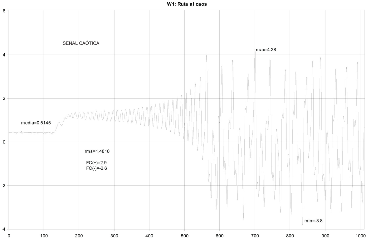
Figura 1. W1: señal caótica (Núñez, 2006) mostrando algunas de sus características: media, valor pico max/min, valor eficaz y sus FC. Se observa el inicio del caos a partir de los 570 m/seg producto de la bifurcación (vertical: voltios, horizontal: m/seg)
