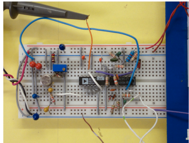
Figura 7. Tablilla de simulación mostrando el CFC en pruebas de validación
