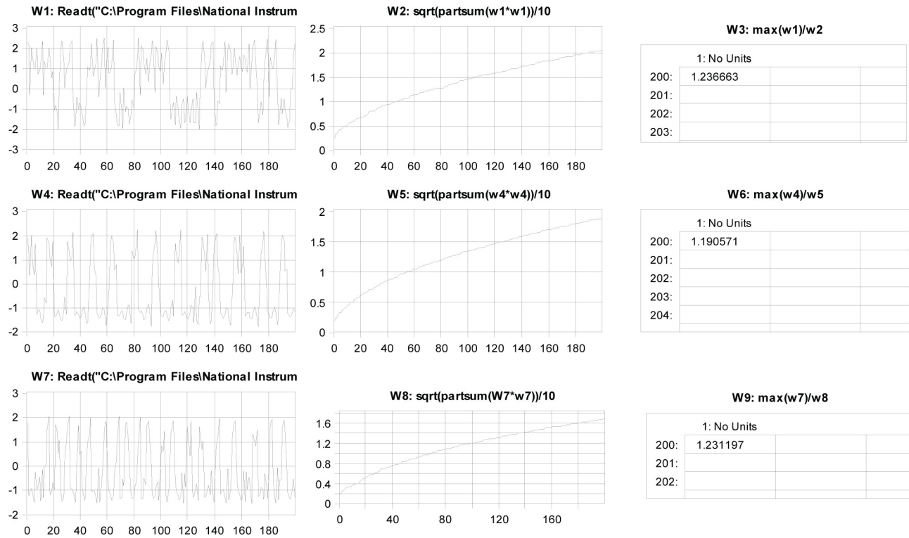
Figura 15. Señales caóticas V \times t del circuito Chua, generadas con parámetros diferentes y cálculo de sus FC asociados utilizando el programa DADISP. Entre más caotización mayor distorsión y la tendencia del FC también aumenta (vertical: voltios, horizontal: m/s)
