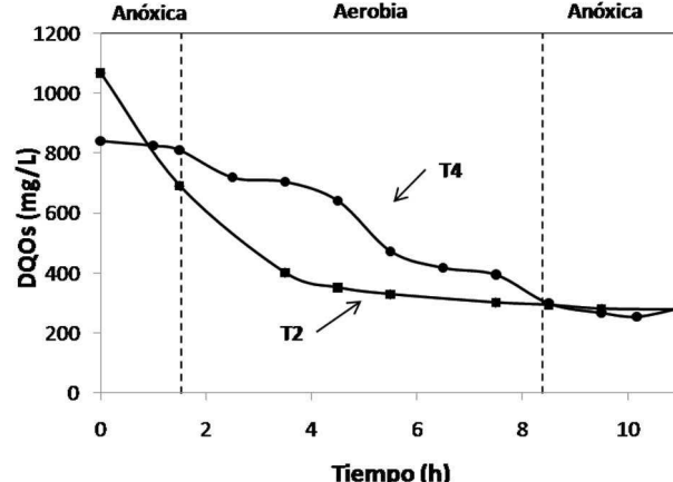
Figura 5. Evolución de la DQO_5 durante un ciclo de operación del SBR para los tratamientos T2 y T4
