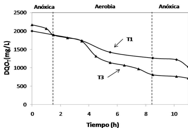
Figura 2. Evolución de la DQO_7 durante un ciclo de operación del SBR para los tratamientos T1 y T3
