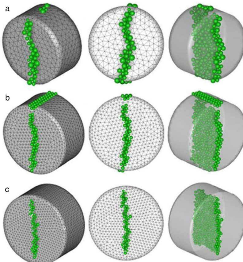
Figura 11. Ensayo de tracción indirecta. Grieta y elementos discretos generados. a) Malla gruesa; b) malla intermedia; c) malla fina.
