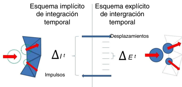
Figura 2. Integración temporal en subetasas utilizado para el análisis conjunto de elementos finitos y discretos.
