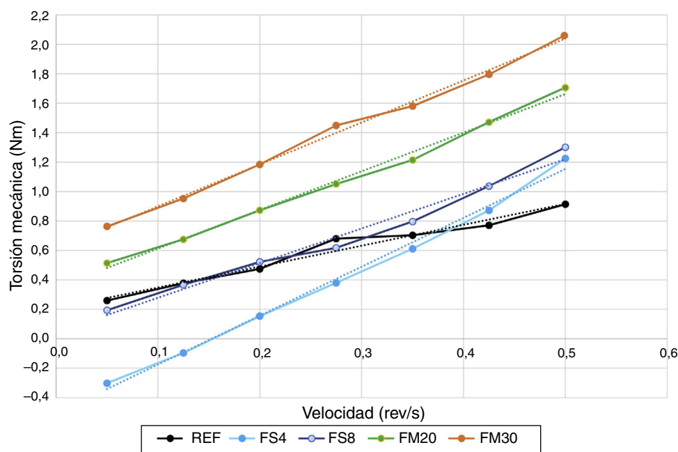
Figura 1. Resultados obtenidos con réómetro rotacional de paletas.
