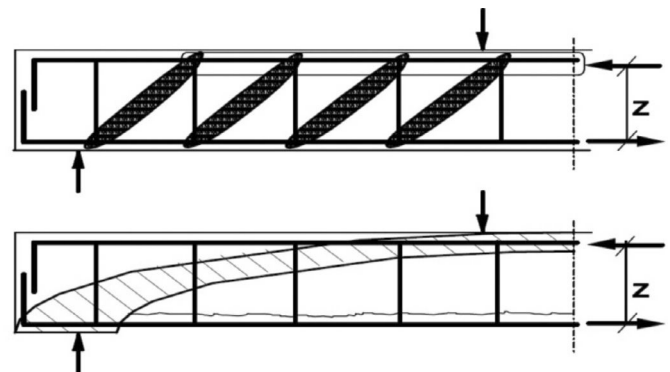
Figura 7. Modelo viga versus modelo arco atirantado en elementos flectados con pérdida de adherencia en zonas intermedias de las barras.
