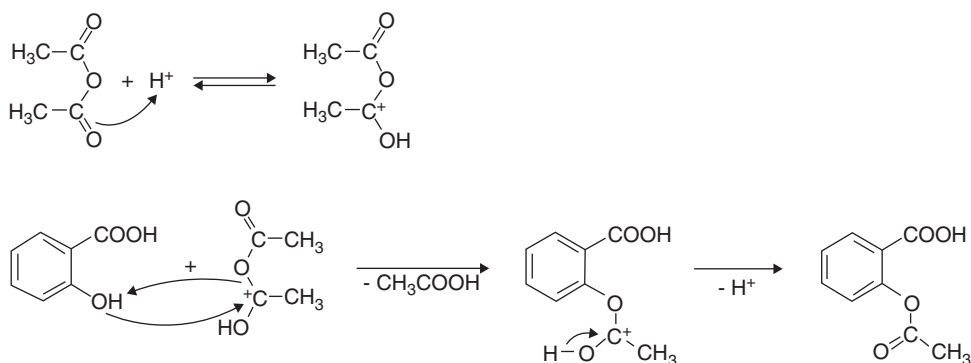
Figura 1 Estructura química de la aspirina.
