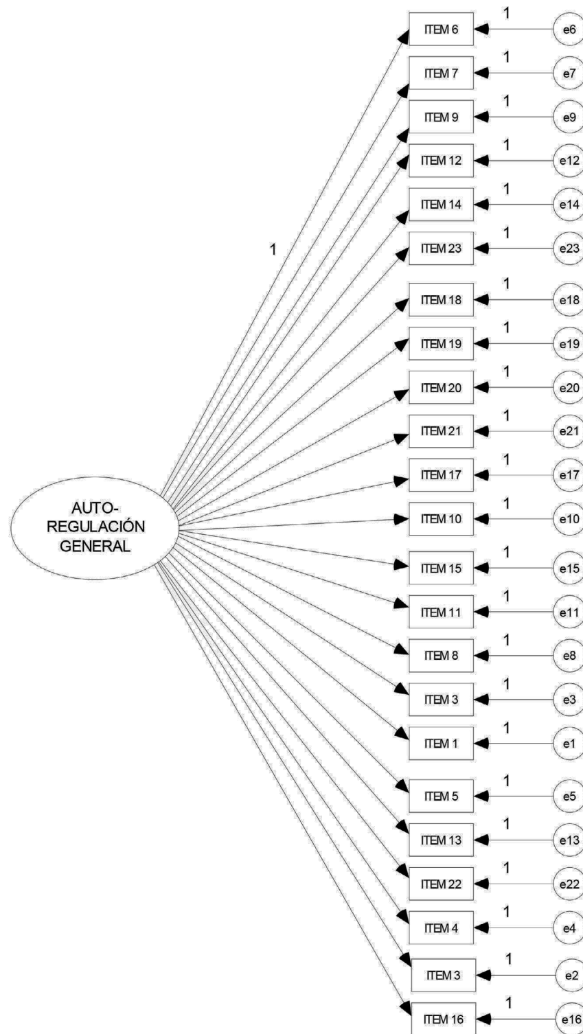
Figura 1 Modelo 1 (un factor general que explica la varianza de todos los ítems de ARATEX-R).
