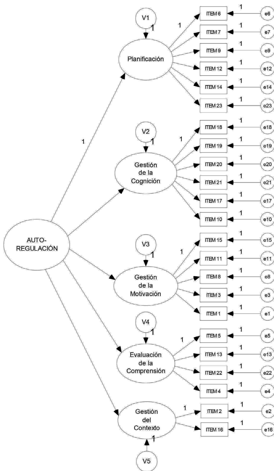
Figura 4 Modelo 4 (modelo de cinco factores de primer nivel, con un factor general de segundo nivel).
