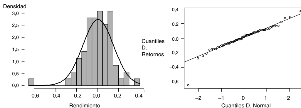
Figura 1. Histograma de rendimientos mensuales y diagrama de probabilidad Normal (Q-Q plot) de la acción GGAL.
