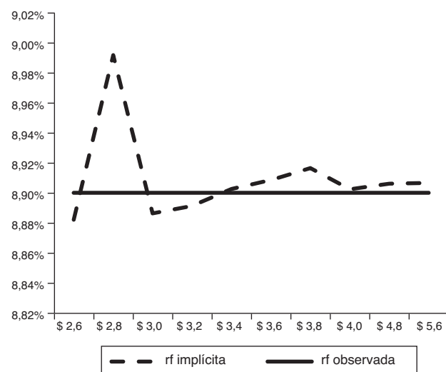
Figura 4. Comportamiento tasa libre de riesgo (rf) implícita y observada. Fuente: elaboración propia.
