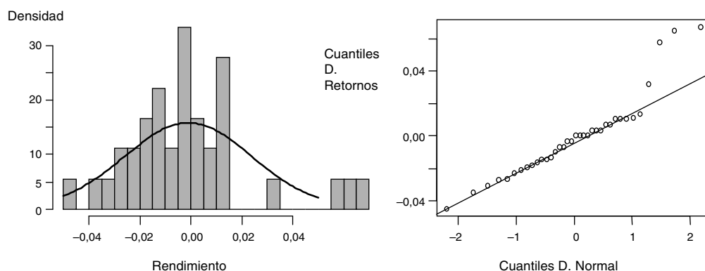
Figura 2. Histograma de rendimientos diarios y diagrama de probabilidad Normal (Q-Q plot) acción GGAL.
