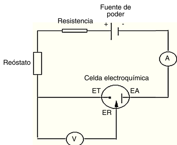
Fig. 2 Esquema del montaje experimental del potenciostato de bajo costo. A: amperímetro; EA: electrodo auxiliar o contrario; ER: electrodo de referencia; ET: electrodo de trabajo; V: voltímetro de alta resistencia.
