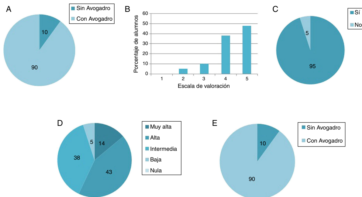
Figura 4 Resultados a las preguntas de la encuesta. Letra A, pregunta 1; letra B, pregunta 2 (1: muy en desacuerdo, 2: en desacuerdo, 3: más o menos, 4: de acuerdo, 5: muy de acuerdo); letra C, pregunta 3; letra D, pregunta 4; letra E, pregunta 5. Todos los valores se presentan en porcentaje.
