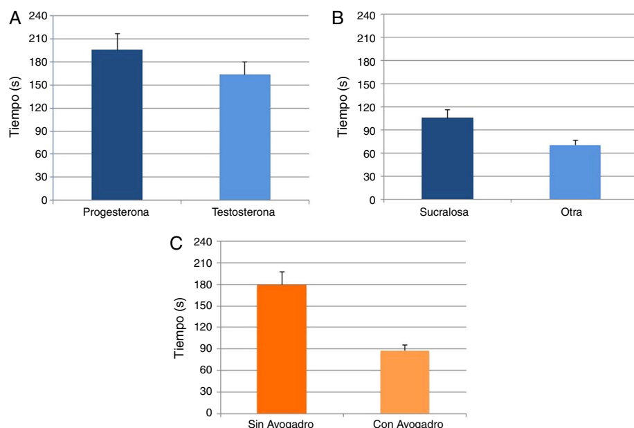
Figura 3 Comparación temporal promedio para la asignación de los carbonos quirales de: 2 esteroides, progesterona y testosterona, A; sucralosa y otra molécula (ibuprofeno o metilfenidato), B; en moléculas bidimensionales (Sin Avogadro ) versus moléculas tridimensionales (Con Avogadro ), C. Todos los gráficos tienen incorporada la desviación estándar normalizada.
