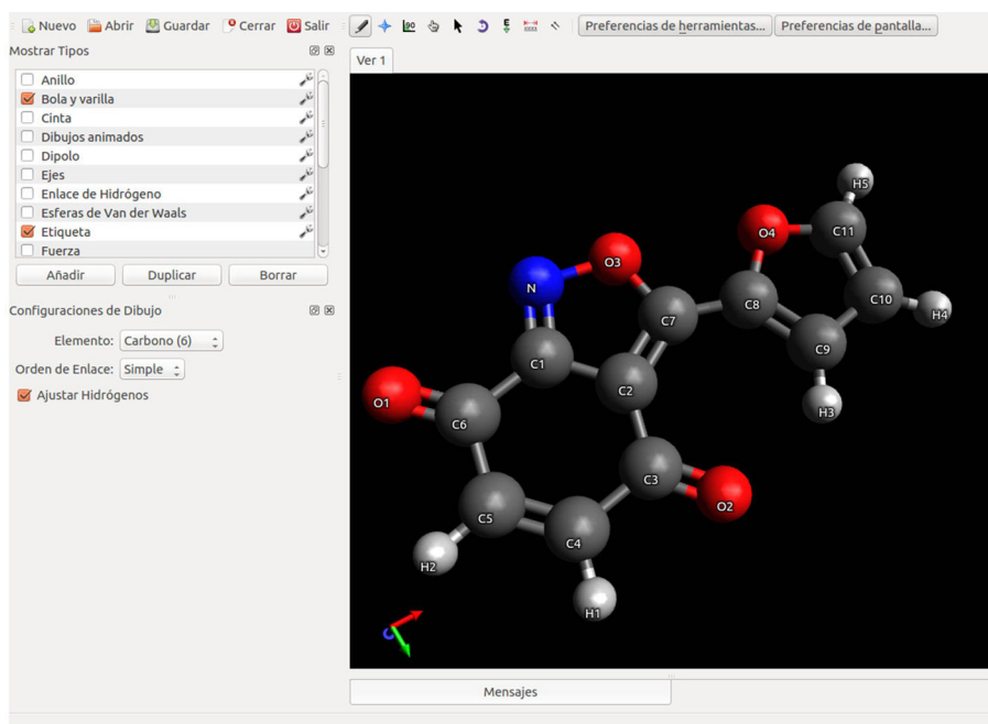
Figura 2 Instantánea del visualizador y constructor molecular Avogadro .
