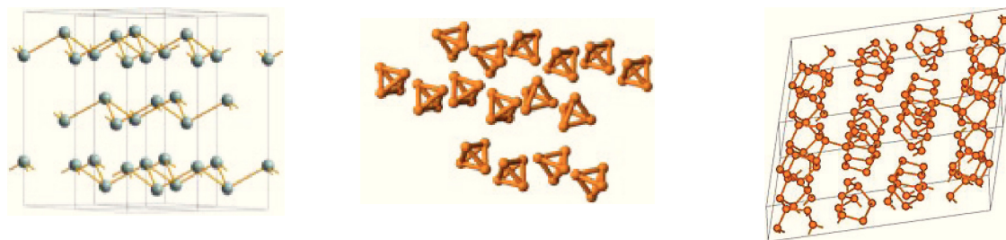
Figura 2. Formas alotrópicas del As y sus estructuras: de izquierda a derecha: gris, amarillo y negro.
