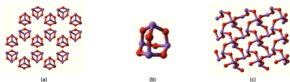
Figura 3. (a) y (b) arsenolita, forma molecular del \text{As}_2\text{O}_3 ; (c) claudetita, forma reticular.
