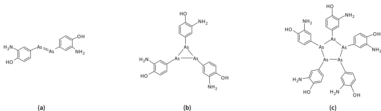
Figura 8. (a) fórmula propuesta por Ehrlich para la arsfenamina; (b) y (c) formas de esta sustancia presentes en el célebre fármaco.
