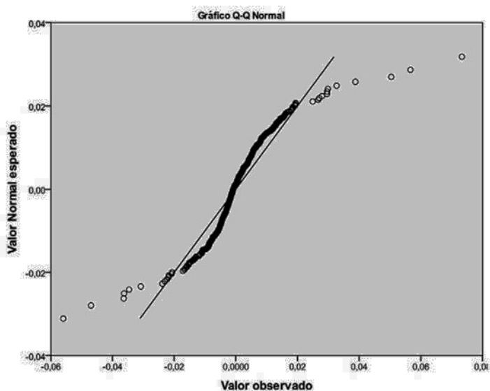
Figura 4 Gráfico Q-Q
