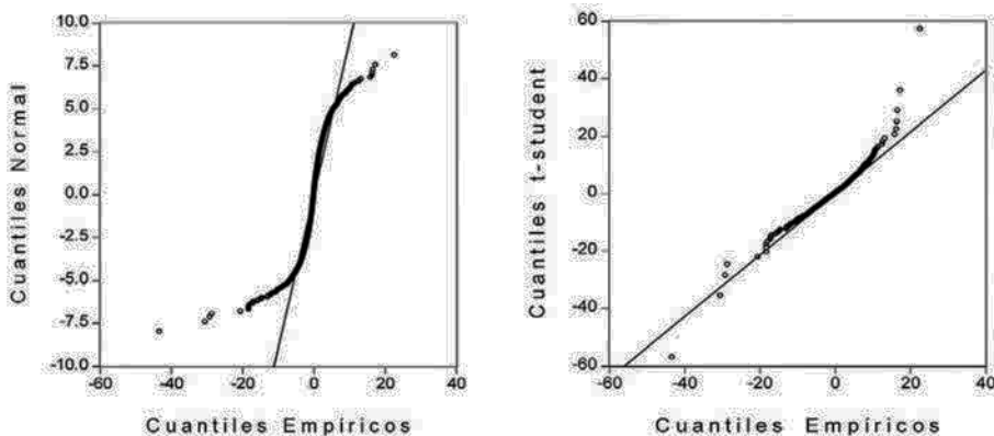
Gráfica 2 Q-Q de los rendimientos diarios contra las distribuciones normal y t-student
