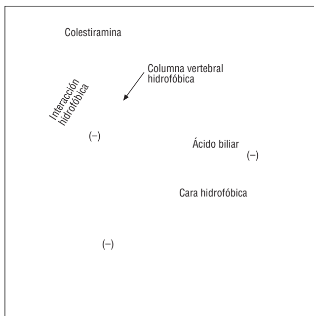
Figura 1 Estructura química de la colestiramina.
