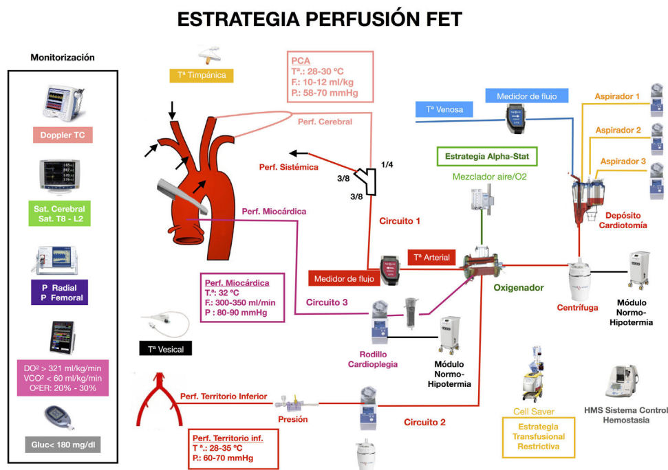
Figura 1. Circuito de TEC a corazón latiendo.
